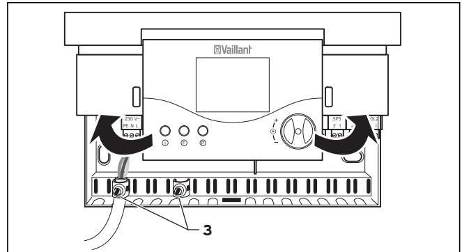
Мал. 4.4 Відкидання органу керування
