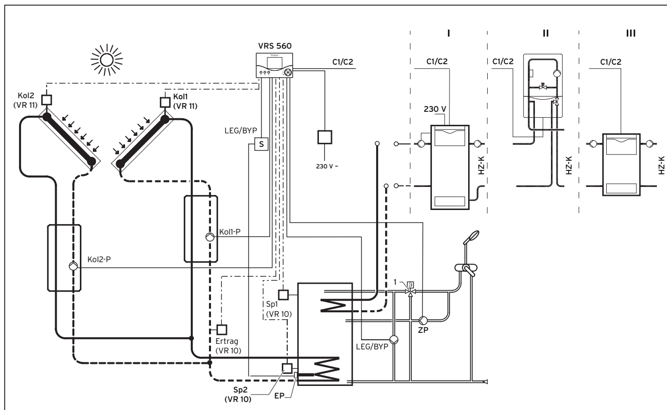
Мал. 5.7 Гідравлічна схема 2 з конфігурацією установки: Дві колекторні панелі, один сонячний накопичувач, можливість підключення різних теплогенераторів для підігріву накопичувача
