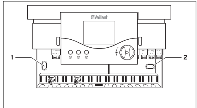
Мал. 4.3 Кріплення корпусу регулятора
