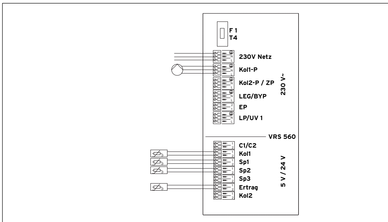
Мал. 5.6 Схема з'єднань для гідравлічної схеми 1: Інтеграція autoMATIC 560 у моновалентну систему
