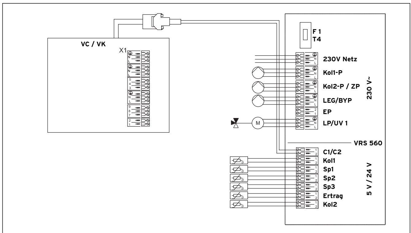
Мал. 5.10 Схема з'єднань для гідрравлічної схеми 2: підключення другого накопичувача або ванни
