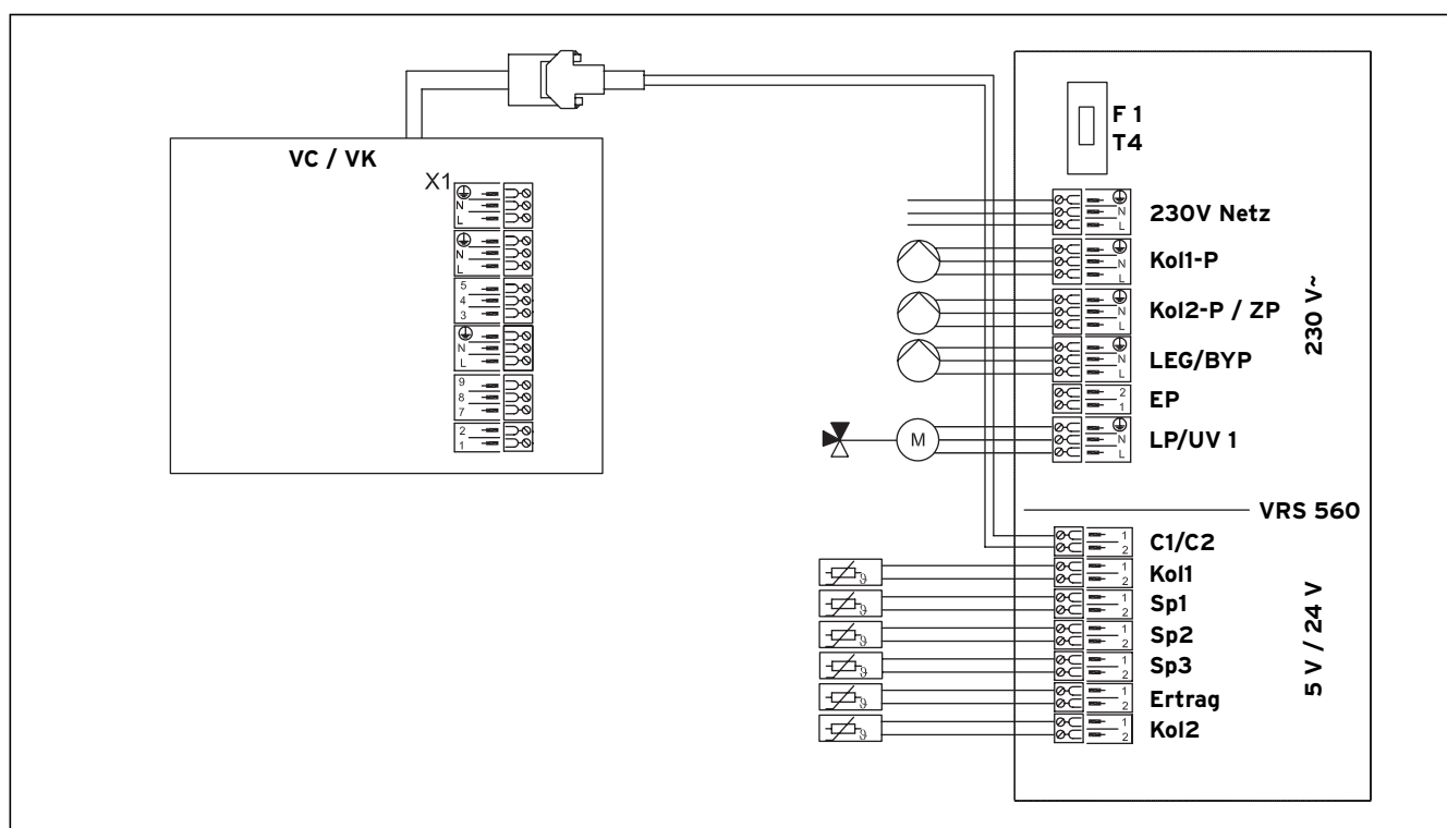
Мал. 5.14 Схема з'єднань для гідрравлічної схеми 3: підключення другого накопичувача або ванни
